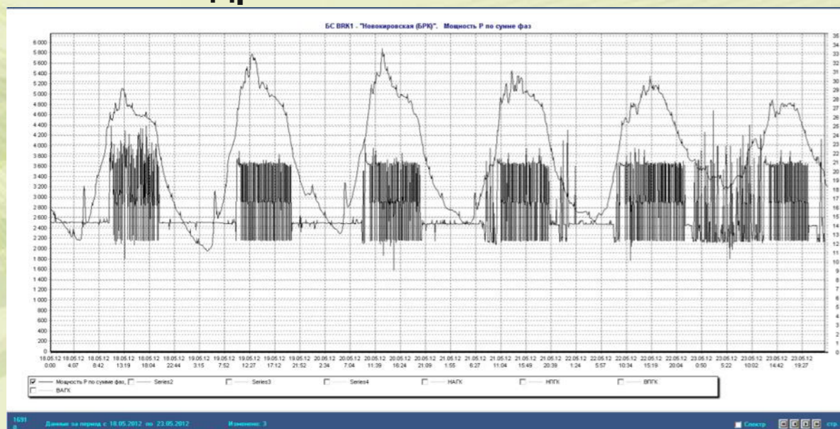
График мощности по сумме фаз после внедрения СКК на основе БРКВ
