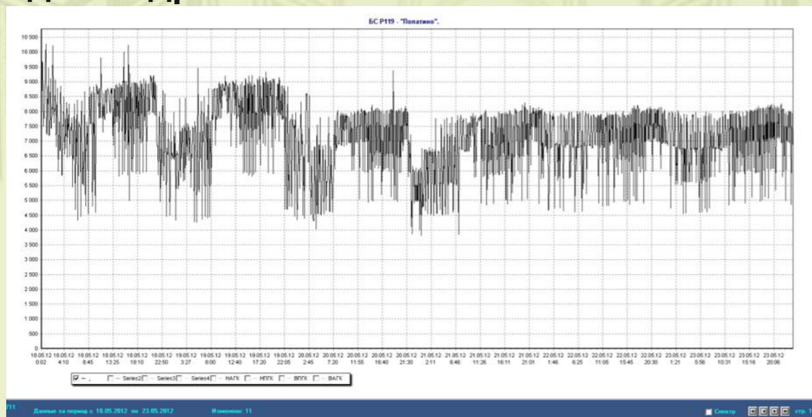
График мощности по сумме фаз до внедрения СКК на основе БРКВ
